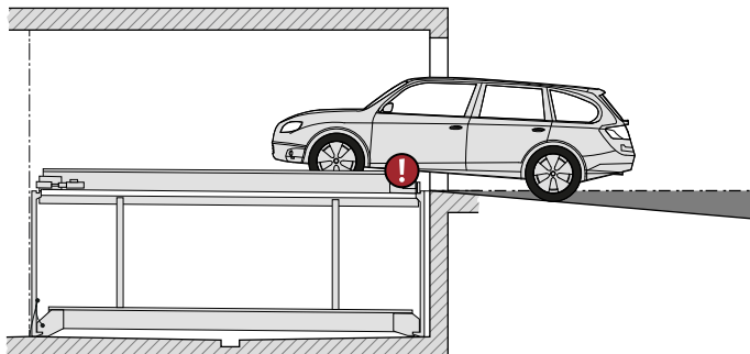
max. 5% gradient
